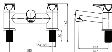
Bath Filler UNDETPBF
