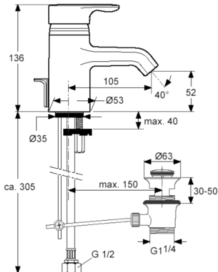
1-Loch Waschtiszbatterie chrom, mit Ab- und Überlaufgarnitur E 6396 AA chrom, ohne Ab- und Überlauf E 6397 AA
