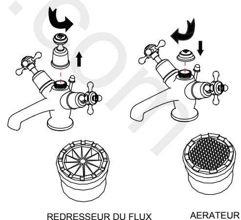
REDRESSEUR DU FLUX
