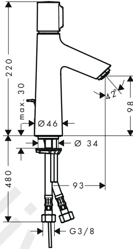
Talis Select S 100 72042000 / 72043000
