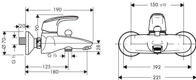
Avista 31748007
