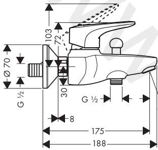
Metropol S 14461007
