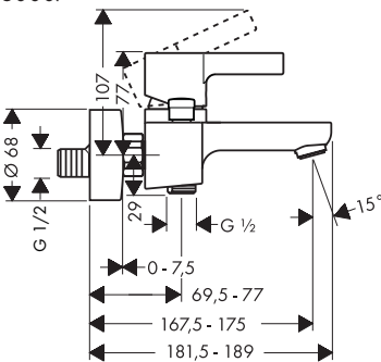
Metris 31480007
