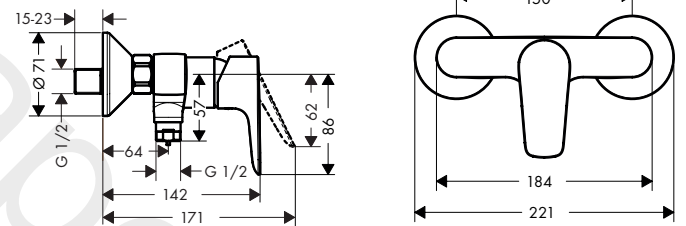
Talis E 71760007
