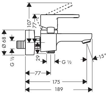
Metropol S 14461007
