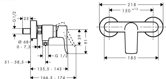
Metris 31680007
