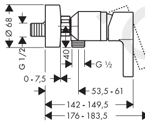
Metris S 31660007
