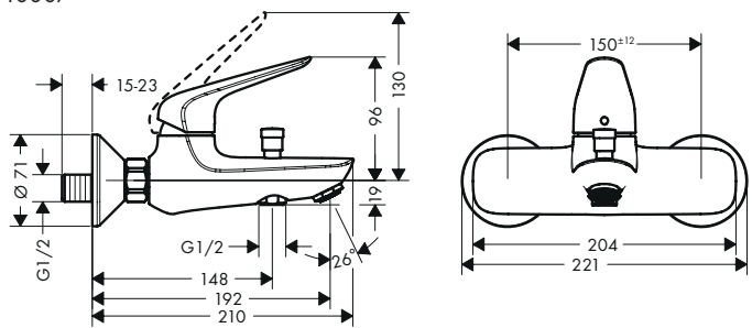
Novus 71040007
