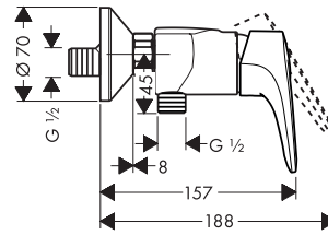
Metropol E 14670007
