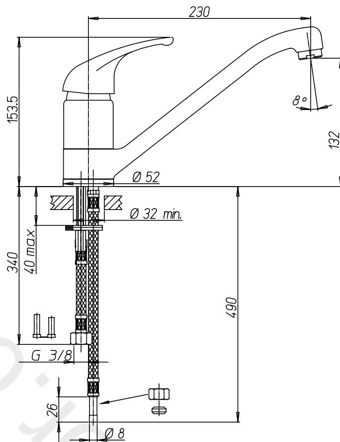
ESEMPIO DI INSTALLAZIONE IDRAULICO EXAMPLE OF INSTALLATION
