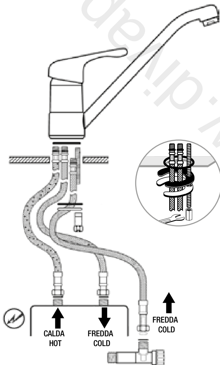
ESEMPIO DI INSTALLAZIONE IDRAULICO EXAMPLE OF INSTALLATION
