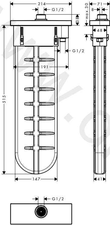
AXOR sBox 28012XXX
