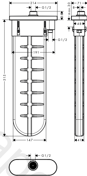
AXOR sBox 28022XXX
