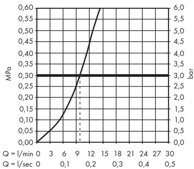
AXOR sBox 28012XXX/28022XXX
