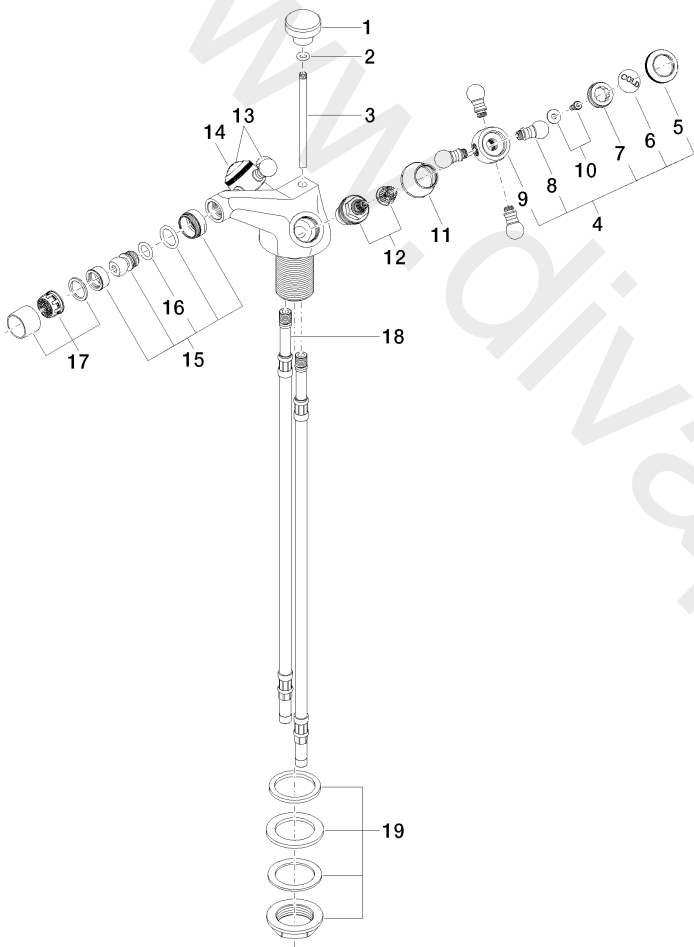
20 — Ablaufgerät 04.11.01.001.00.fr
