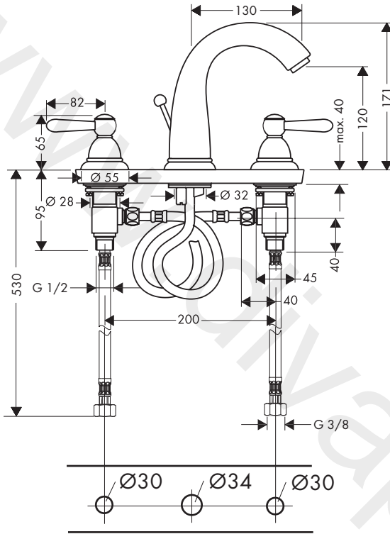
AXOR Carlton 17134XXX
