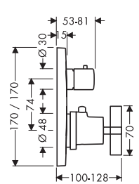
AXOR Citterio 39725000
